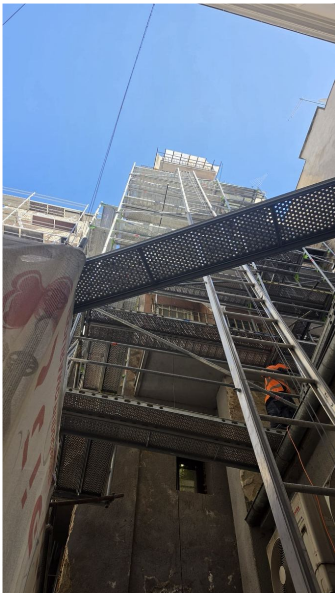
Fasadna skela — ojačanje vanjske konstrukcije
